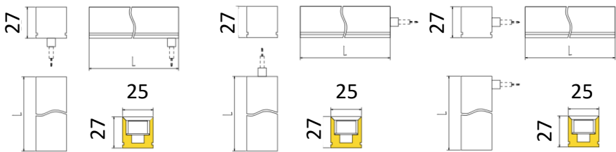
Bottom Outlet
