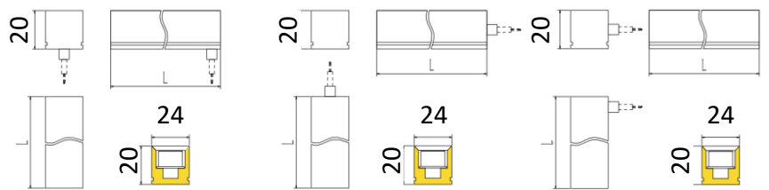
Bottom Outlet
